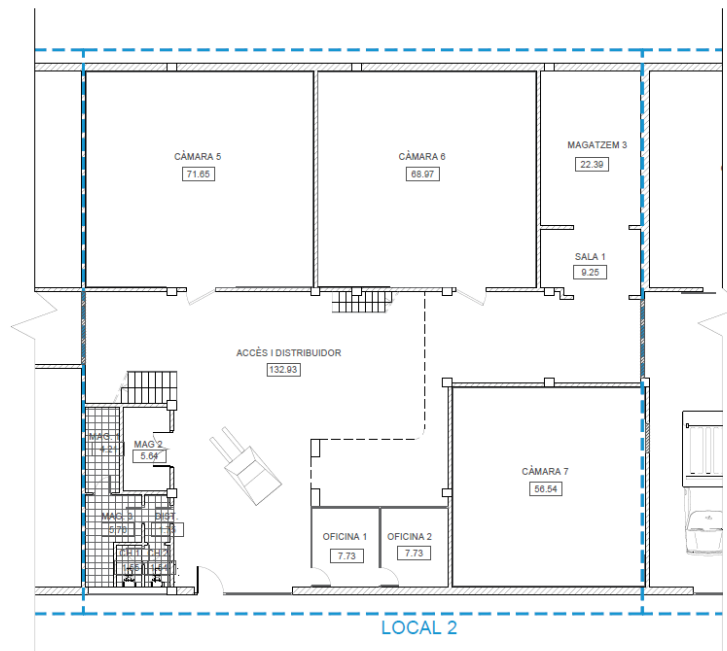
PLANTA BAIXA
