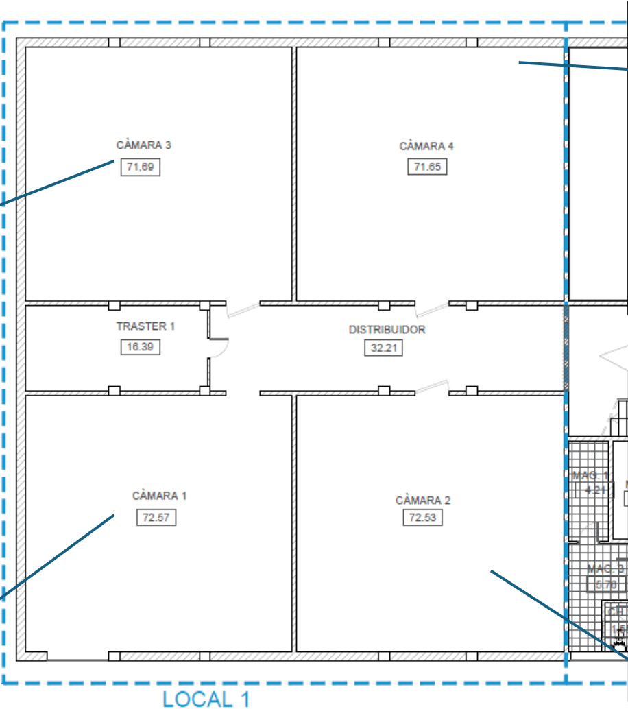
PLANTA BAIXA
